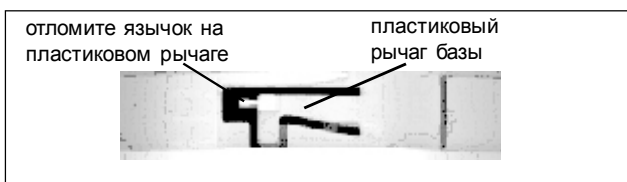
Рис. 4. Активизация функции защиты от несанкционированного извлечения извещателя
