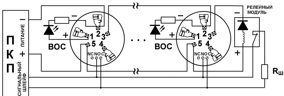
Рис. 2. Типовая 4-х проводная схема подключения базовых оснований B412NL к ПКП (контакты релейного модуля показаны при включенном напряжении питания)
