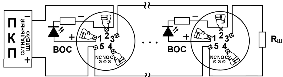
Рис. 3. Типовая 2-х проводная схема подключения базовых оснований B412NL к ПКП
