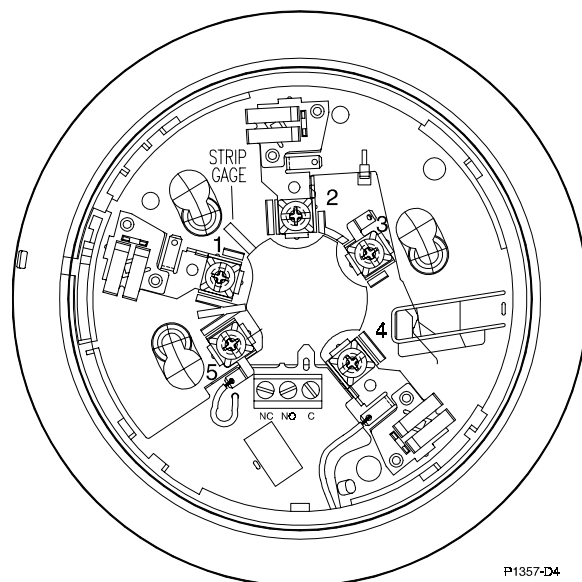
Рис.1 Расположение контактов базового основания В412NL
