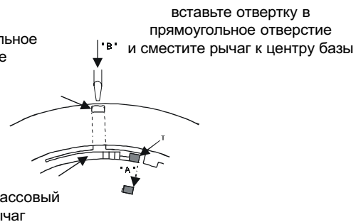
Рис. 5. Извлечение извещателя из базы после активизации защиты
