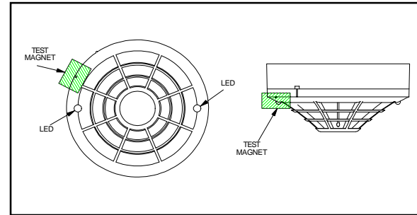
Abbildung 2. Positionieren des Testmagneten
