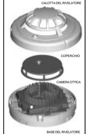
Figura 3: Rivelatore Combinato Ottico Termico 2351TEM
