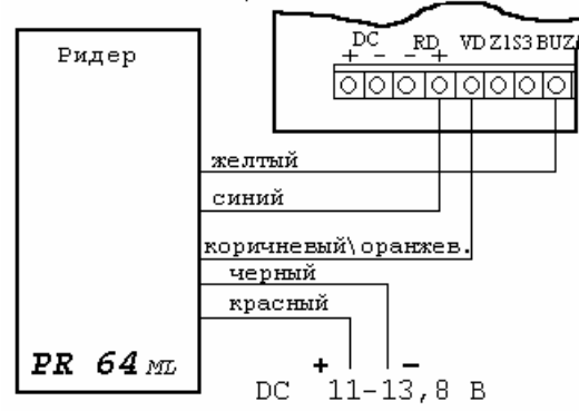
Схема подключения к MD64S, MD256, MD1024
