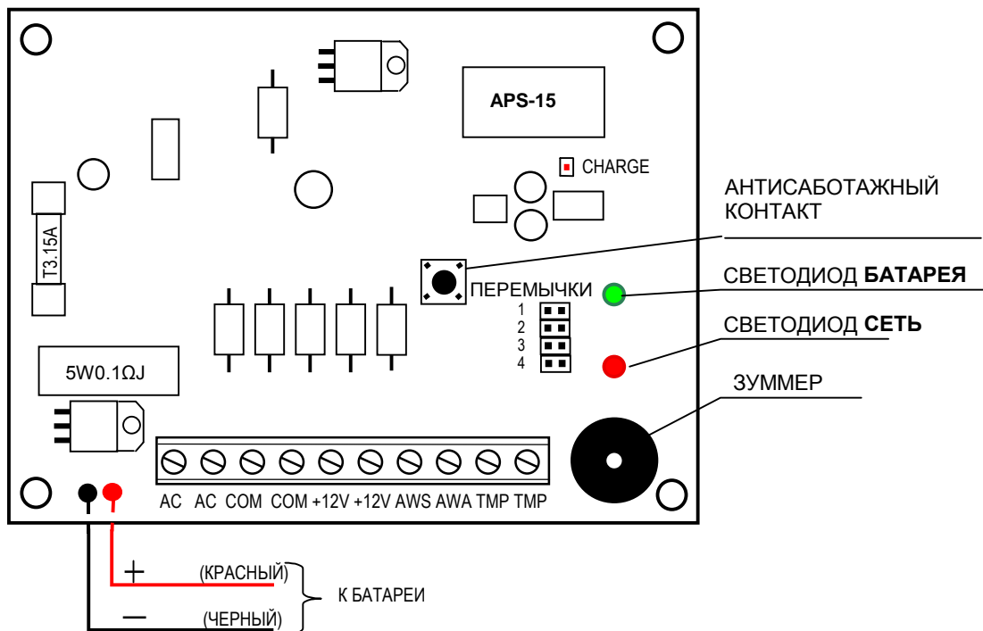
Рис . 1. Плата блока питания с зажимами.
