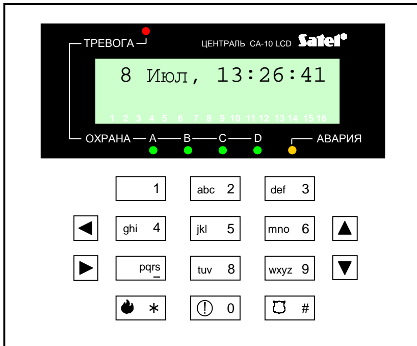
Рис. № 1 - Общий вид панели манипулятора CA-10 KLCD-S
