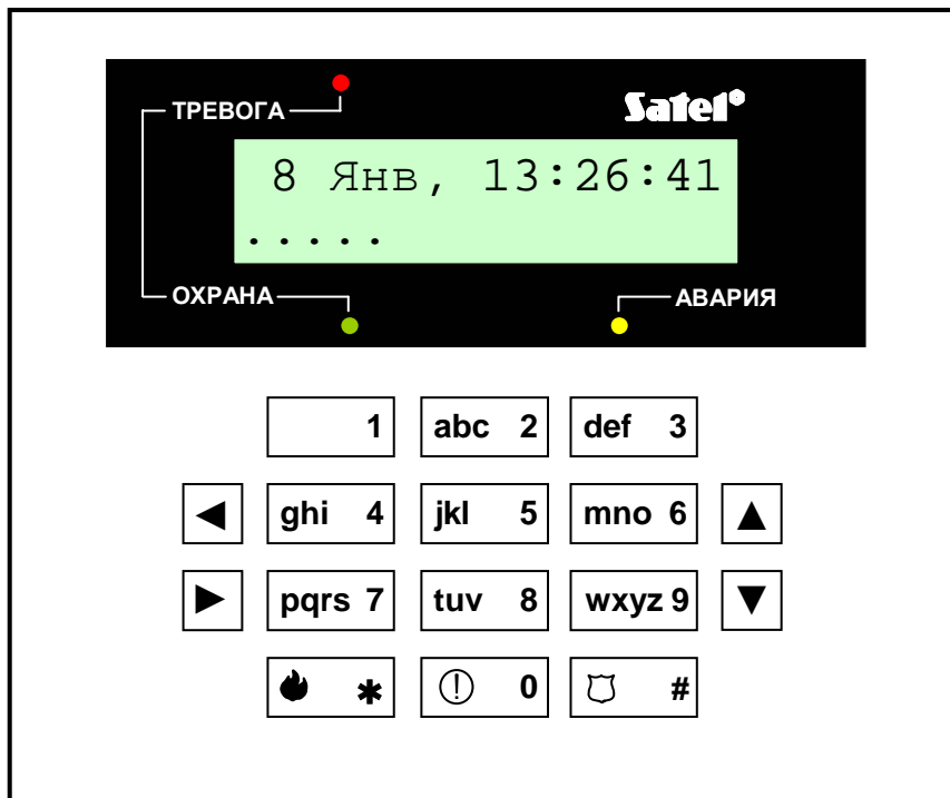
Рис. № 2. Манипулятор типа LCD.
