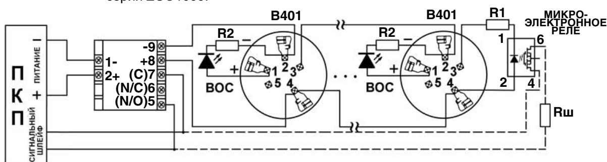
Рис. 2. Схема подключения УС к ПКП и к базам B401 с извещателями 2151E, 5451E.
