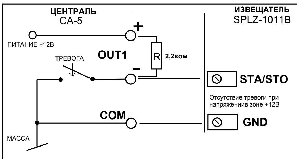
Рис. № 2: Схема подключения извещателя к выходу типа „общее питание” в центральях CA-4V1 и CA-5.
