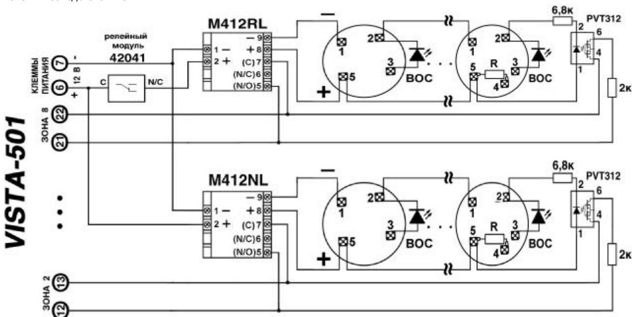
Рис. 4. Схема включения извещателей серии ECO1000 в шлейфы зон 2 - 8 через модули согласования M412RL, M412NL по 2-х проводной схеме
