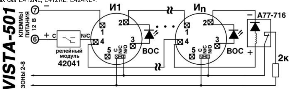
Рис. 3. Схема включения извещателей серии ECO1000 с 4-х проводными базами E412NL, E412RL, E424RL в шлейфы зон 2 - 8
