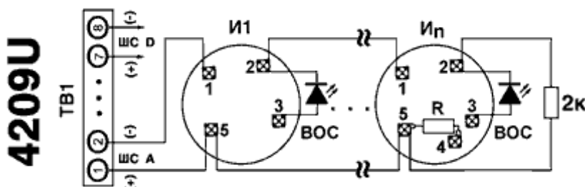
Рис. 2. Схема включения извещателей серии ECO1000 в шлейф адресного расширителя 4209U
